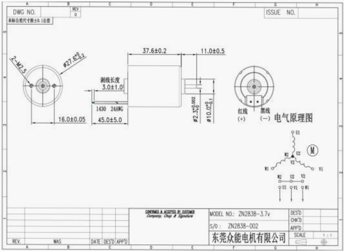
尺寸图 \ Dimension drawing
